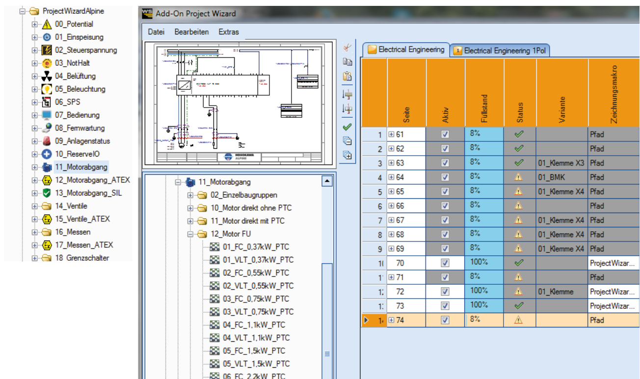
Den größten Teil ihrer Schaltpläne generieren die Entwickler und Konstrukteure bei Hosokawa Alpine schnell über eine Tabelle in dem Add-On Project Wizard der E-CAD-Software WSCAD.
